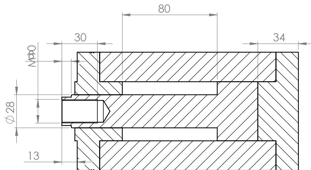
ŘEZ D-D
