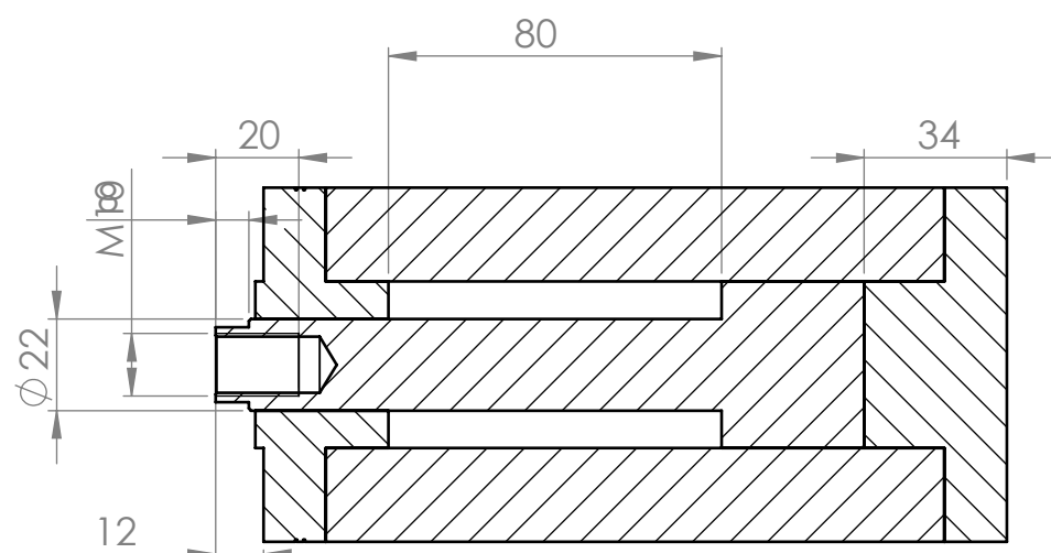
ŘEZ D-D
