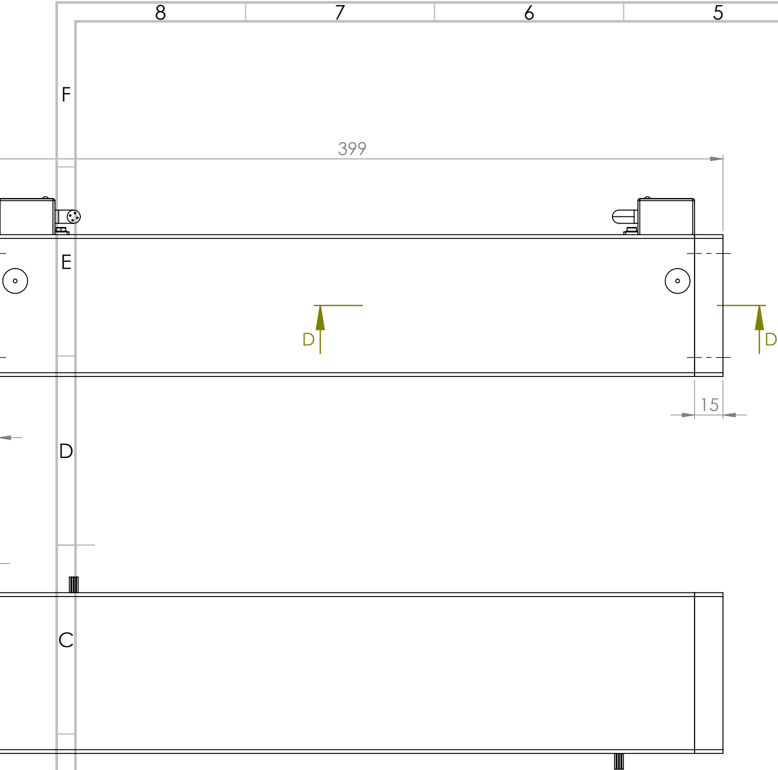
ŘEZ D-D
