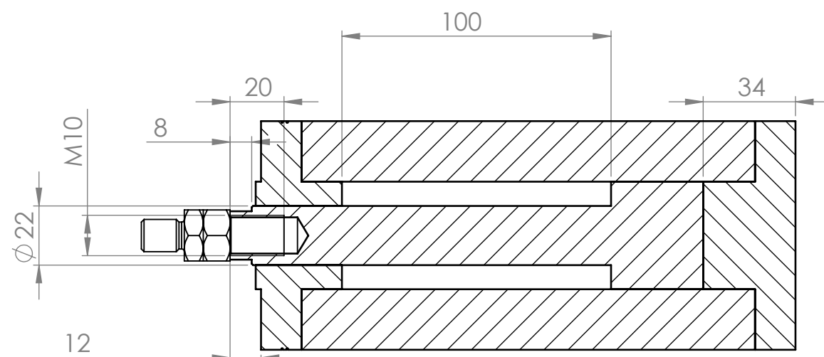
ŘEZ D-D
