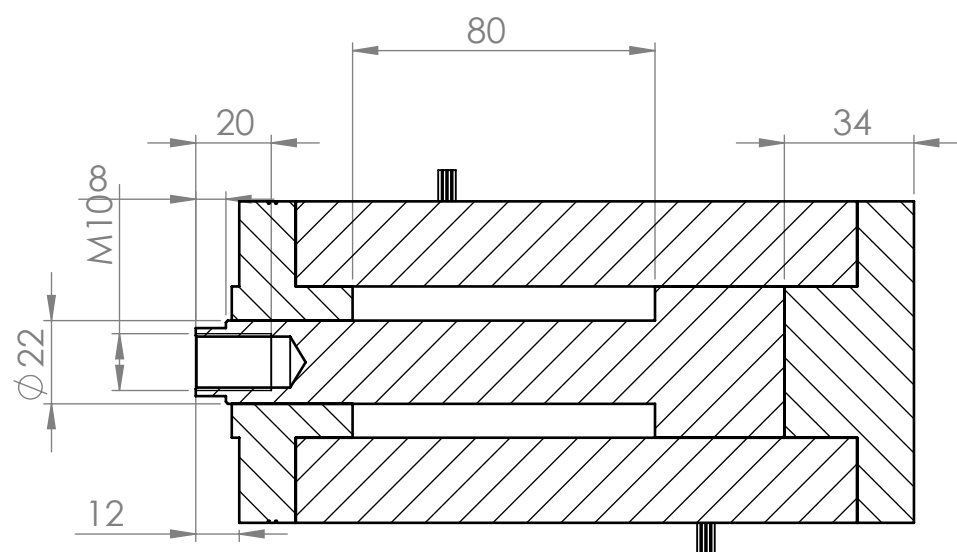
ŘEZ D-D
