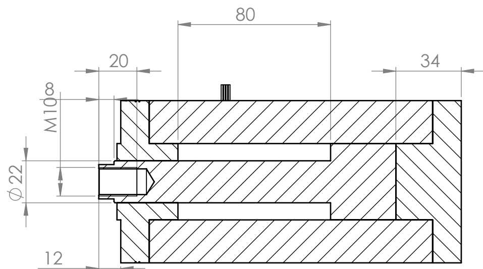
ŘEZ D-D
