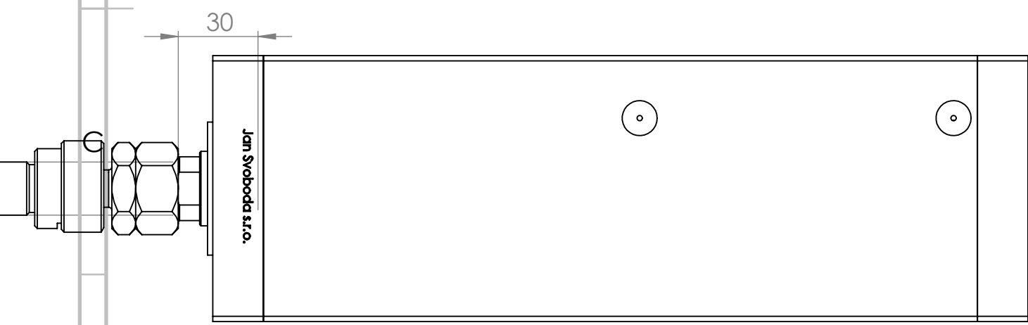
ŘEZ D-D
