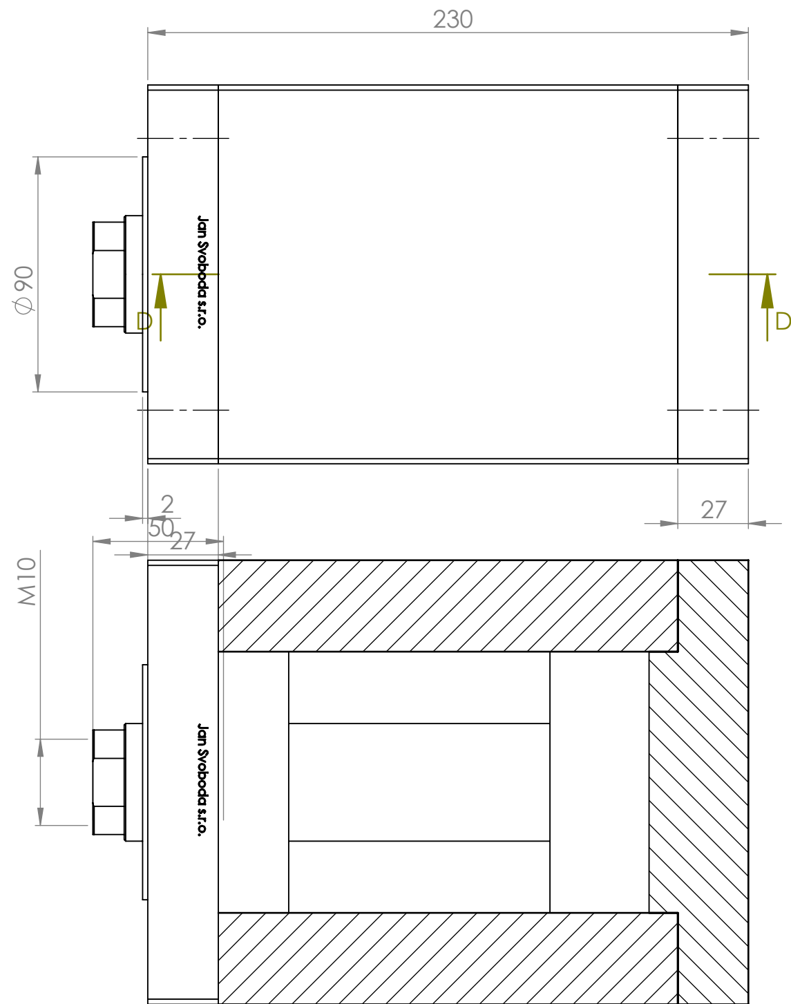
ŘEZ D-D
