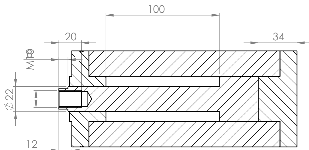
ŘEZ D-D
