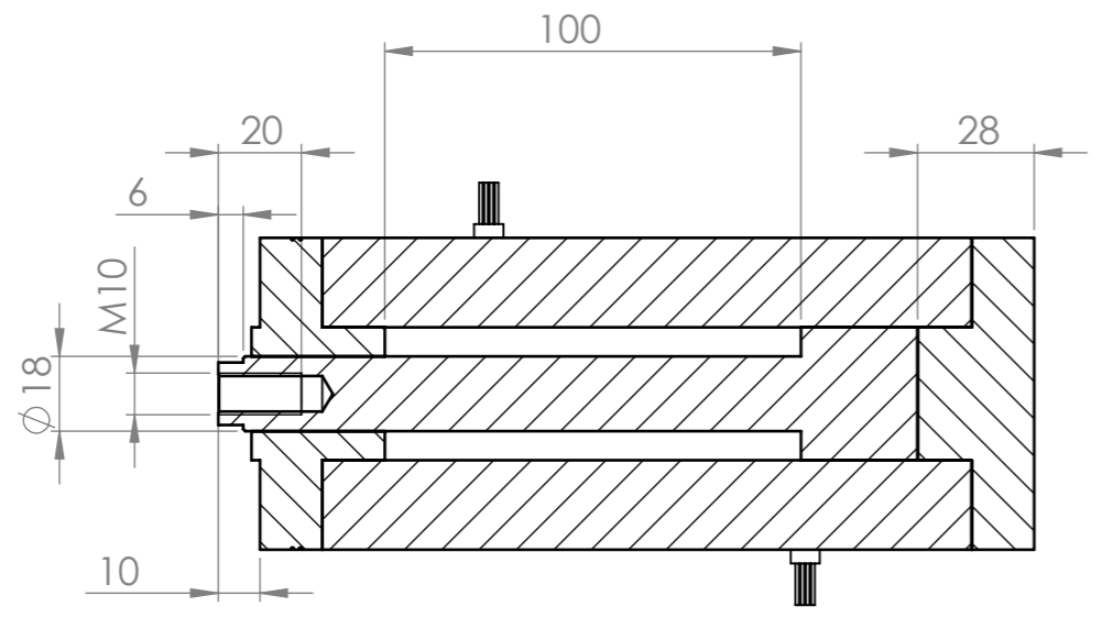
ŘEZ D-D
